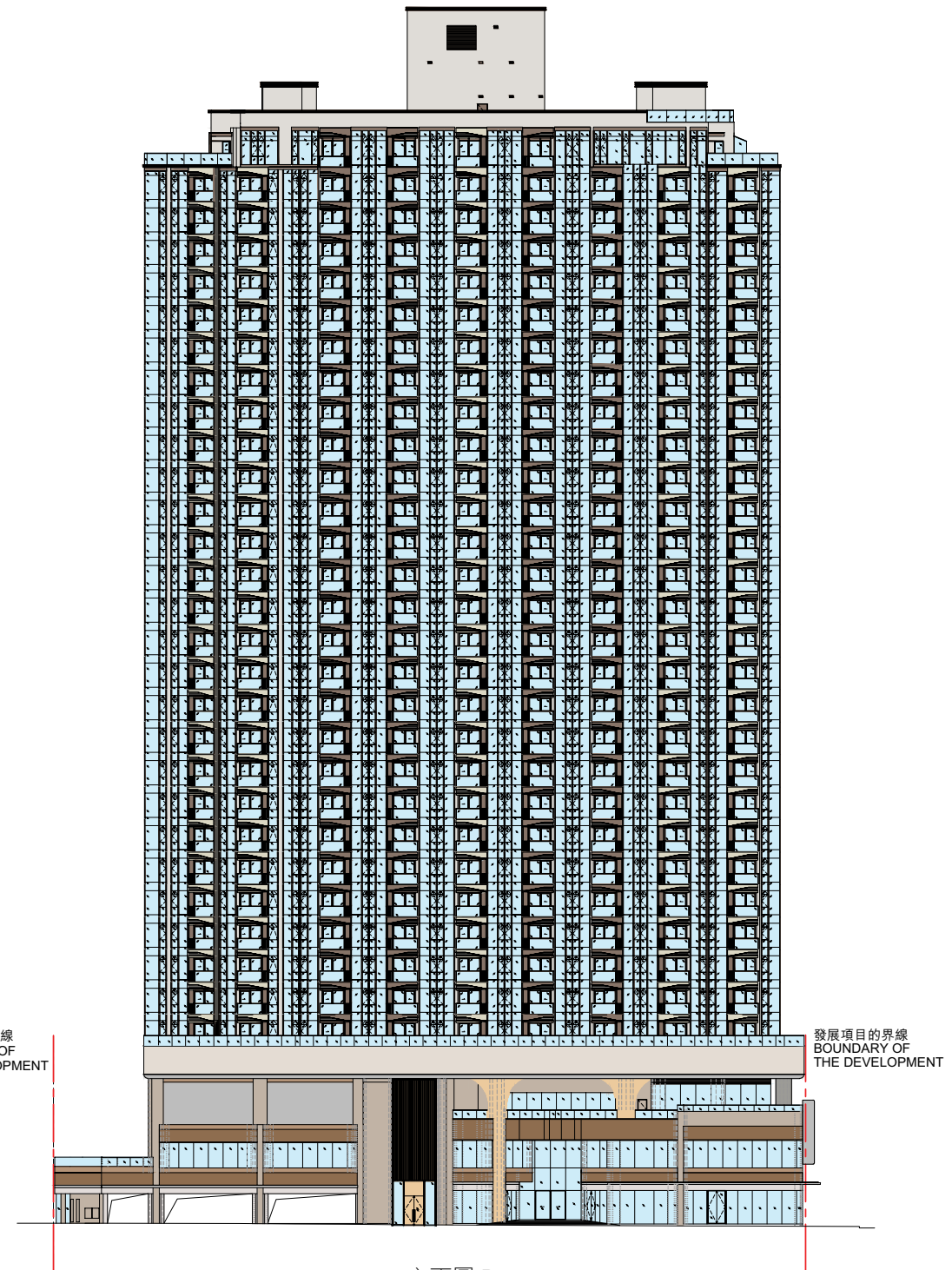
立面圖 D ELEVATION PLAN D
