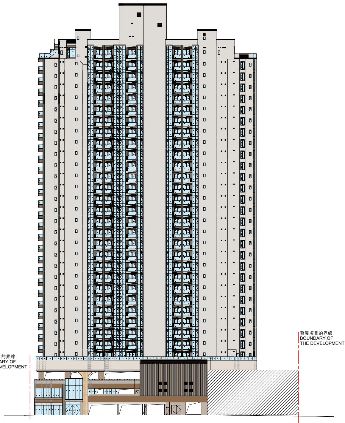
立面圖 B ELEVATION PLAN B
