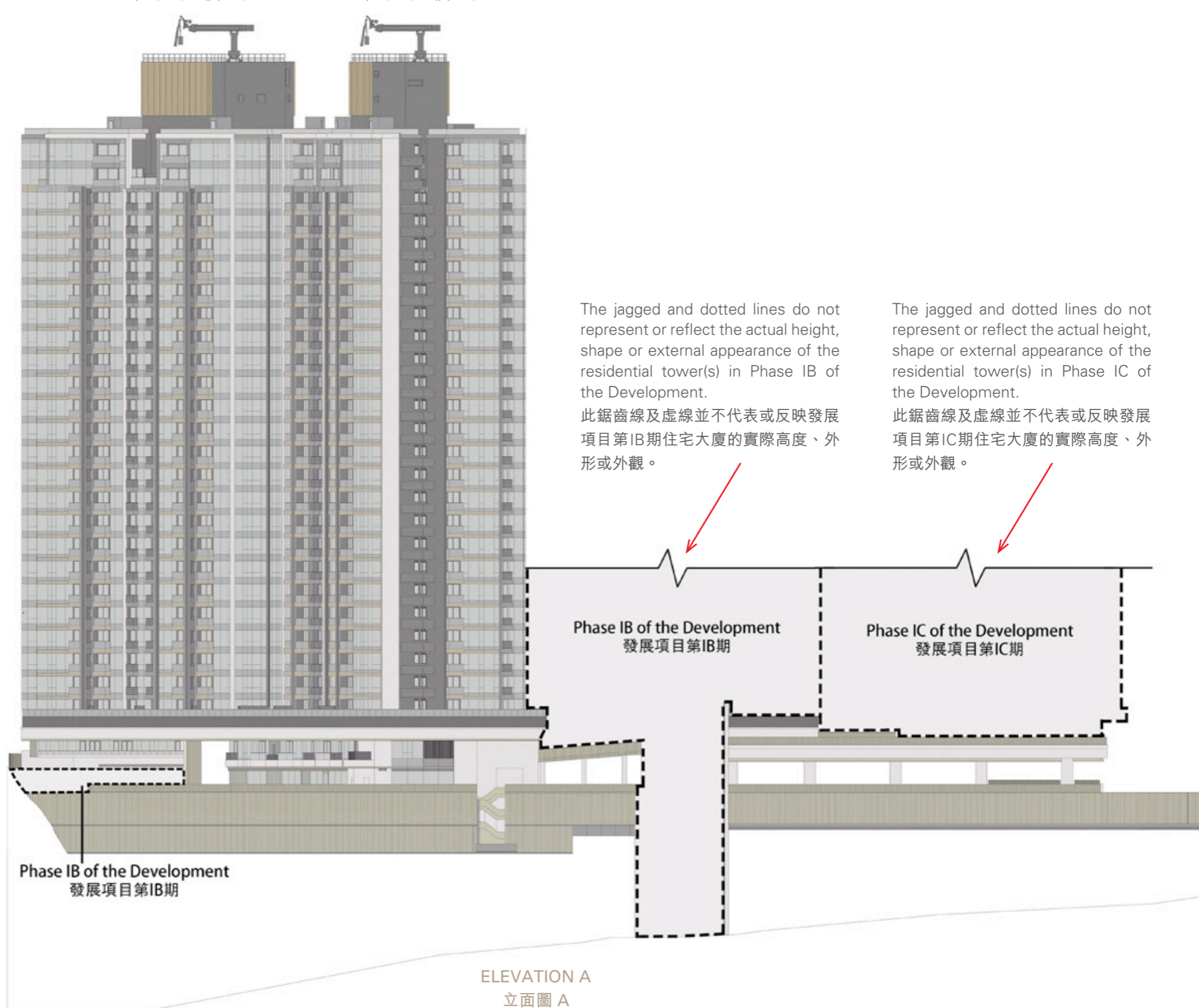
TOWER 2 (2A & 2B) 第2座 (2A及2B)
