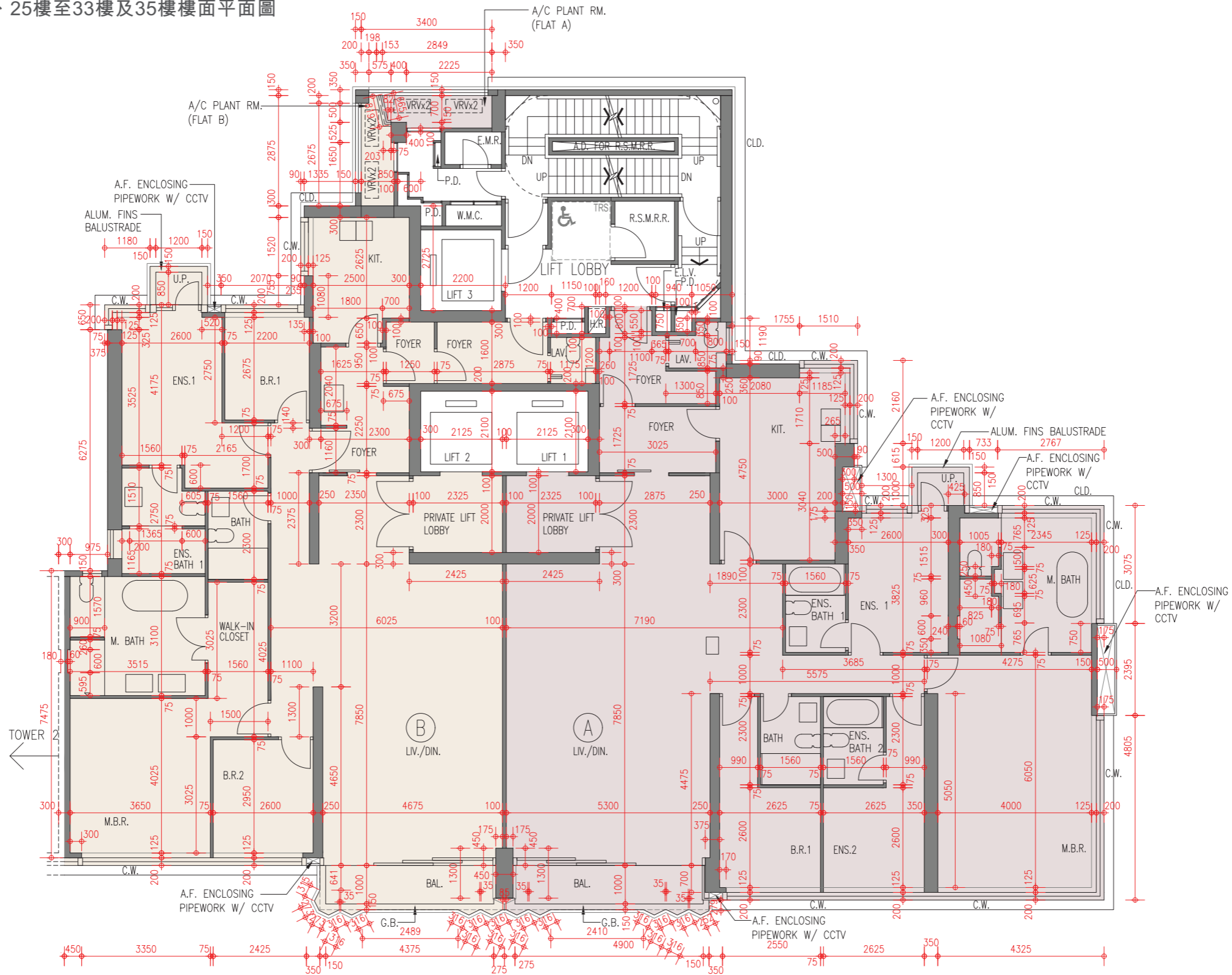
Tower 1 第1座 22/F-23/F, 25/F-33/F & 35/F Floor Plan 22樓至23樓、25樓至33樓及35樓樓面平面圖
