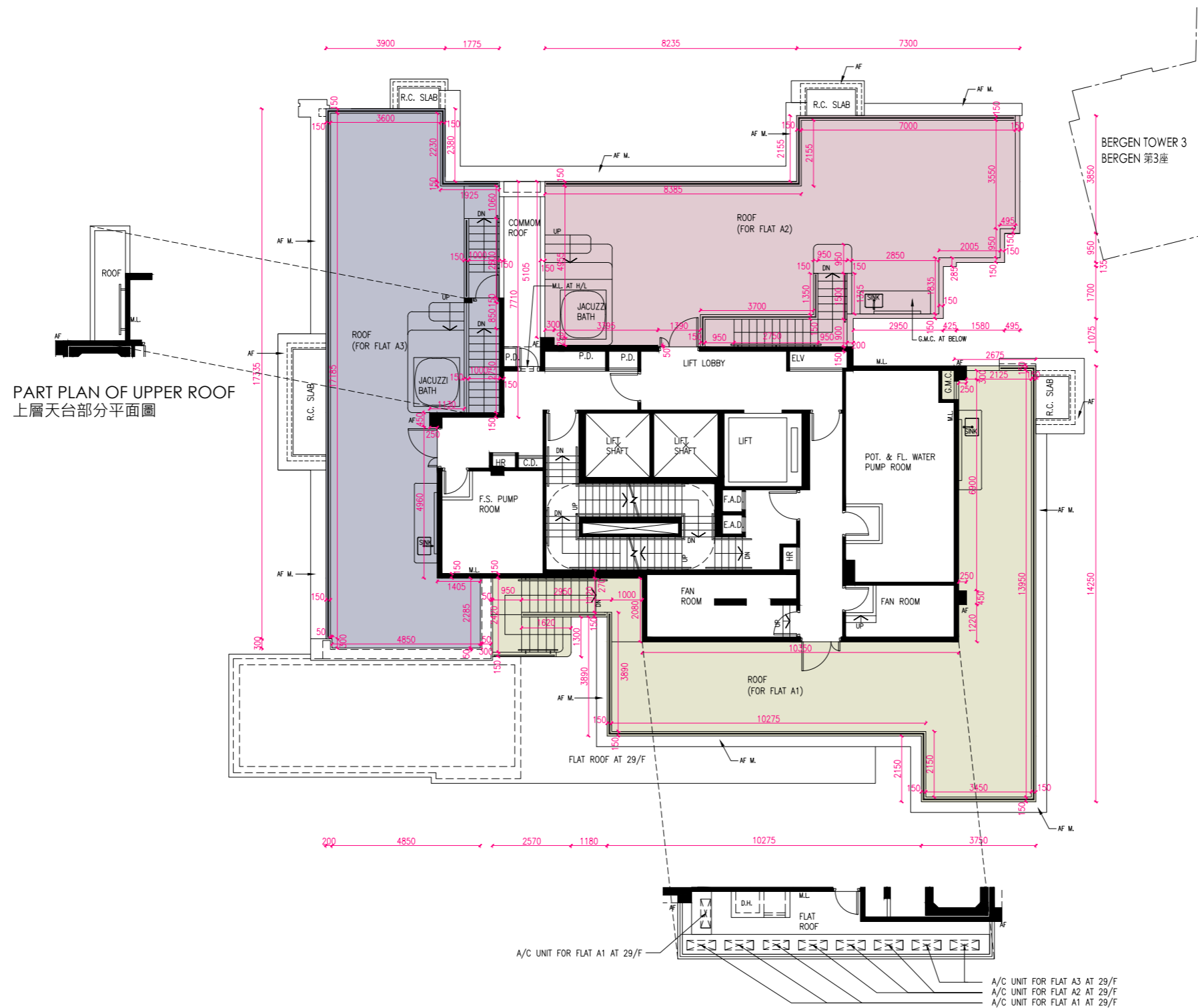
PART PLAN OF UPPER ROOF 上層天台部分平面圖
