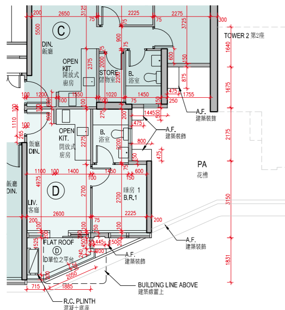
Tower 1 2/F Part Plan 第1座 2樓 局部平面圖
