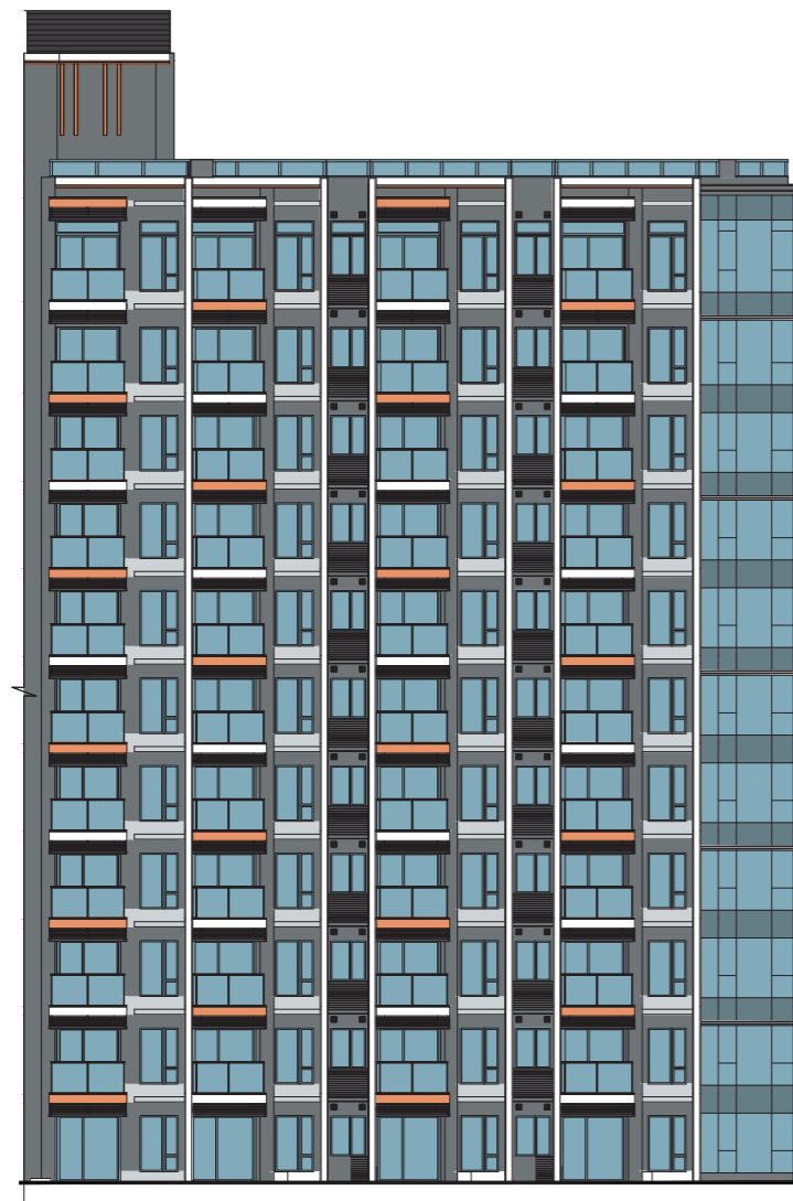
ELEVATION 5 立面 5
