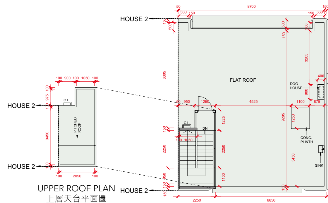
ROOF PLAN 天台平面圖
