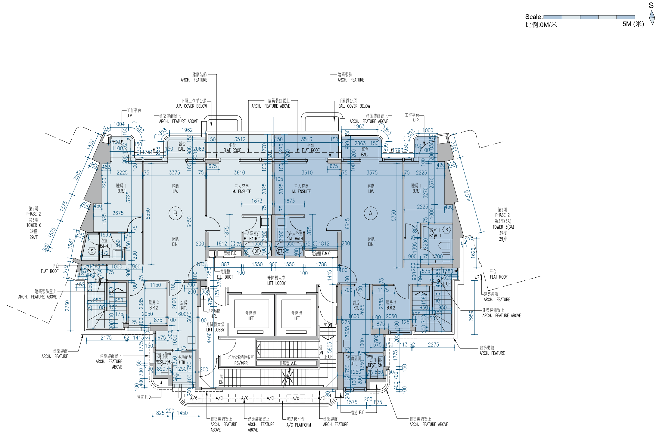
Phase 2 Tower 5 29/F Floor Plan 第2期第5座 29樓樓面平面圖
