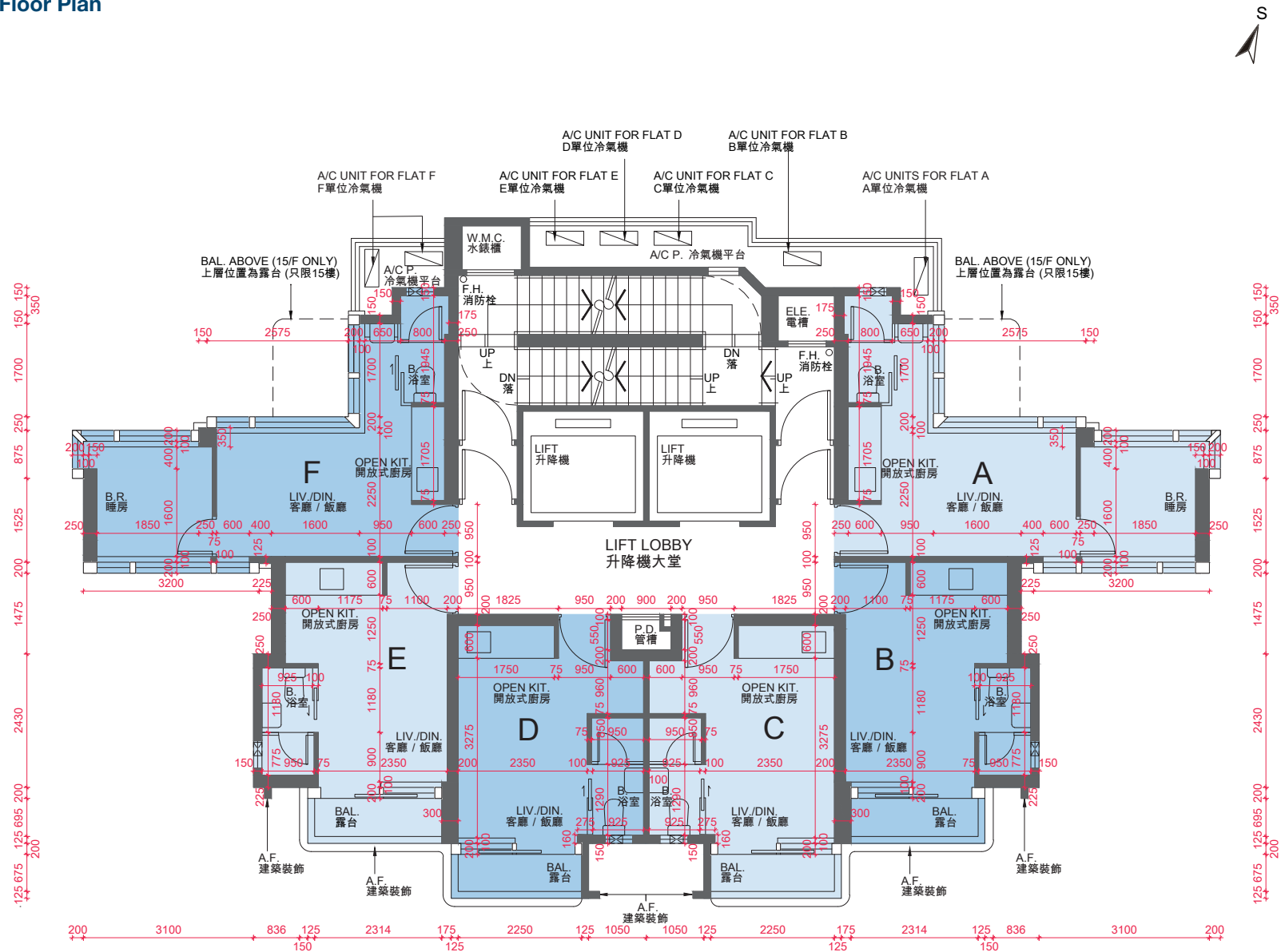
5樓-12樓、15樓平面圖 5/F-12/F, 15/F Floor Plan
