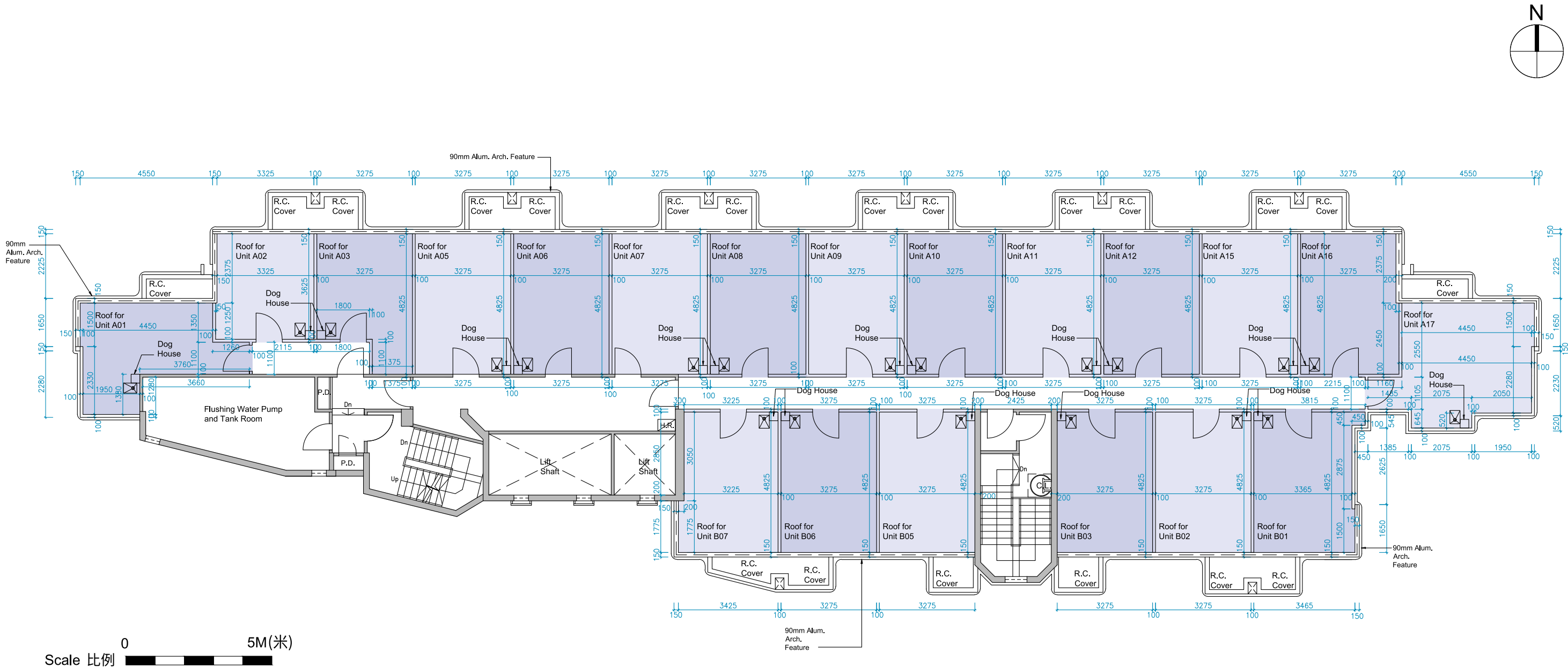
Main Roof Floor Plan 天台平面圖
