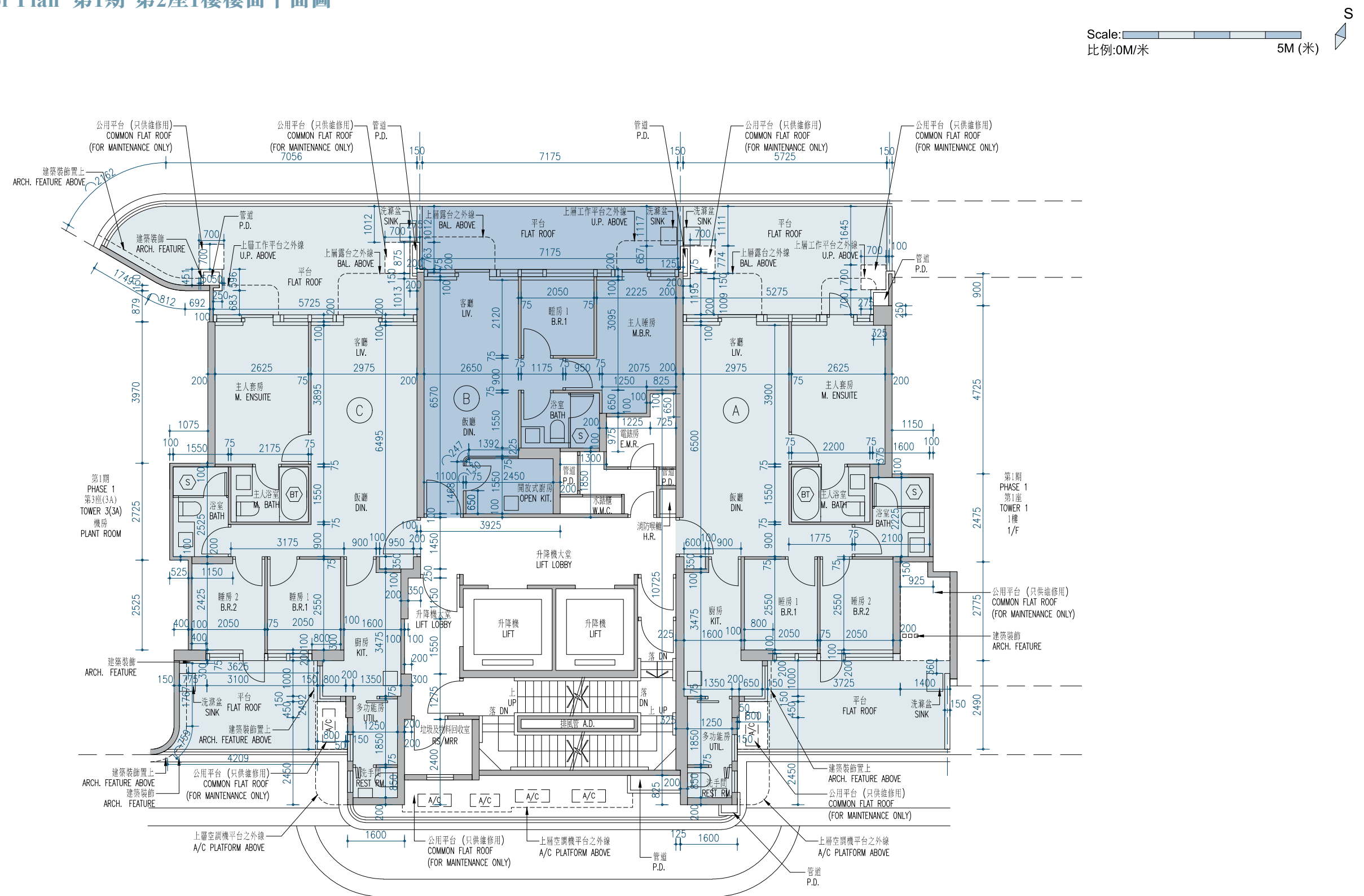
Phase 1 Tower 2 1/F Floor Plan 第1期 第2座1樓樓面平面圖
