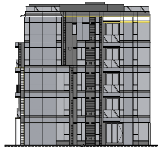
Elevation 2 立面圖2
