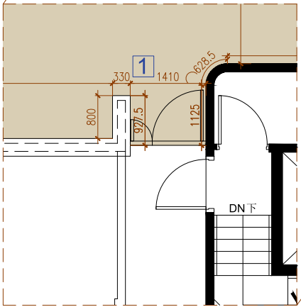
AS-IS PART PLAN OF ROOF 天台現狀部分平面圖
