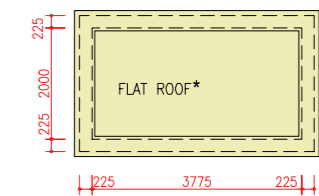
TOP ROOF PLAN 頂層天台平面圖
