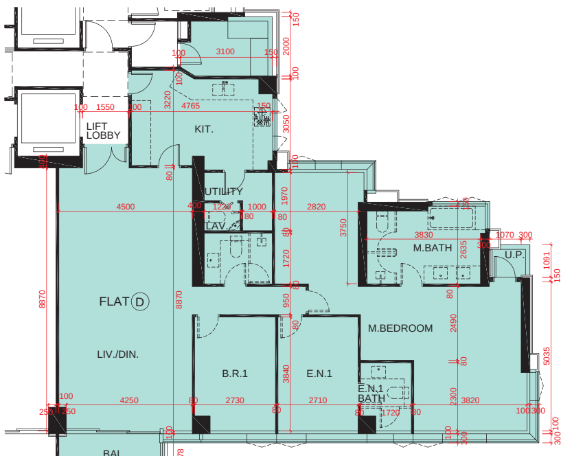
1/F FLAT D FLOOR PLAN 1樓單位D平面圖
