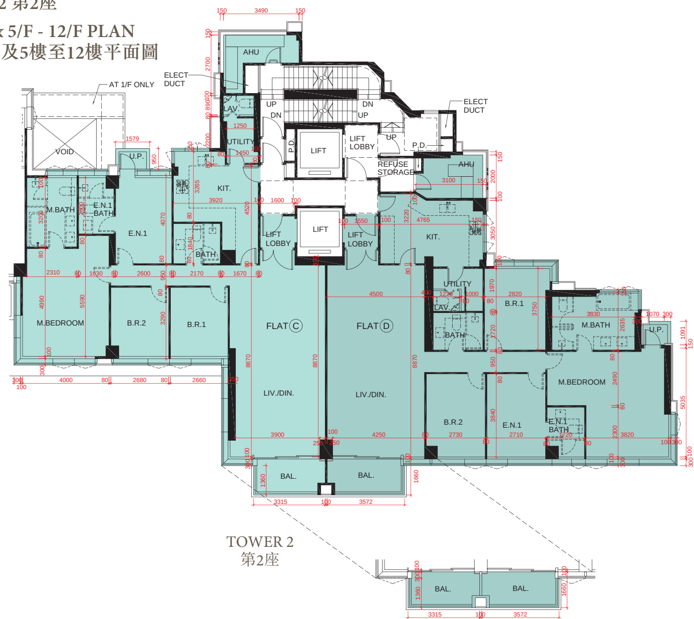
PART PLAN OF 12/F FLAT C & D 12樓單位C及單位D部分平面圖
